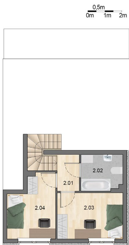
POZIOM 1
