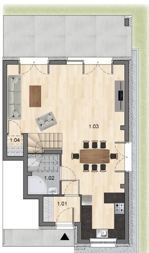
POZIOM 0
